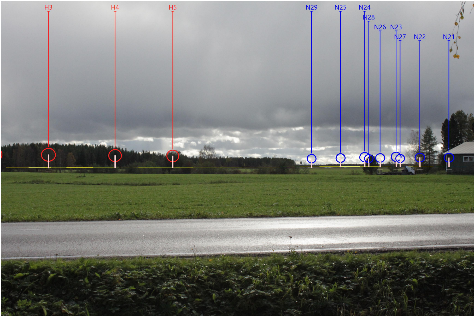
Tuulivoimaloiden sijoittumisen rautalankamalli, pyörähdysala ja numerointi.
