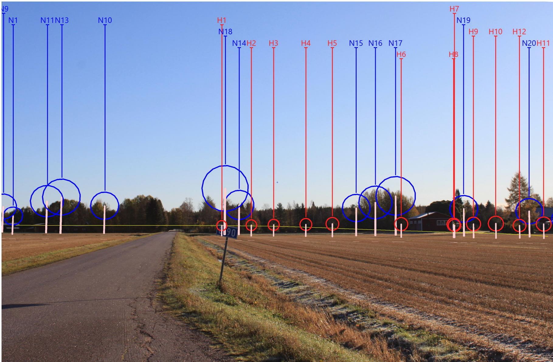
Tuulivoimaloiden sijoittumisen rautalankamalli, pyörähdysala ja numerointi.
