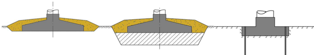
Kuva 82. Tuulivoimalat voidaan perustaa useilla eri tavoilla. Periaatekuvat maanvaraisesta teräsbetoniperustuk-sesta, teräsbetoniperustuksesta massanvaihdon kanssa sekä kallioankkuroidusta teräsbetoniperustuksesta.
