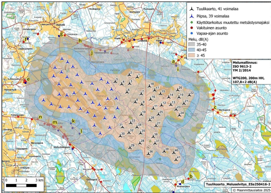
Kuva 75. Melumallinnus yhdessä Piipsannevan voimaloiden kanssa.
