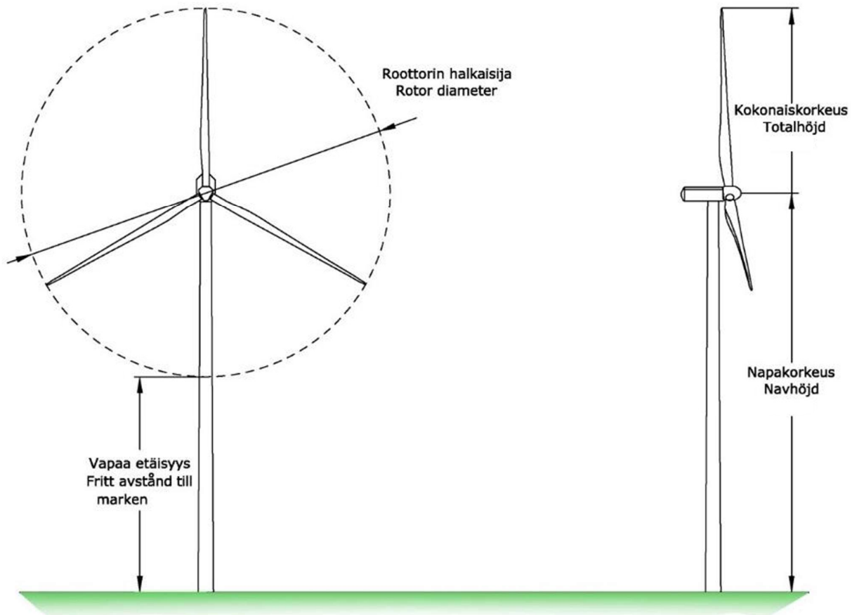
Kuva 79. Tuulivoimalan mallikuva.
