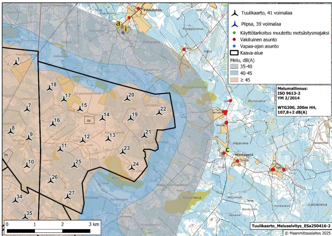
Kuva 76. Yhteisvaikutusten melumallinnus. Siikalatva itäinen kaava-alue.
