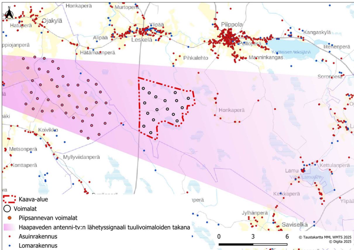
Kuva 65. Haapaveden antenni-tv:n lähetyssignaali Piipsannevan ja Siikalatva itä-kaavan voimaloiden takana.
