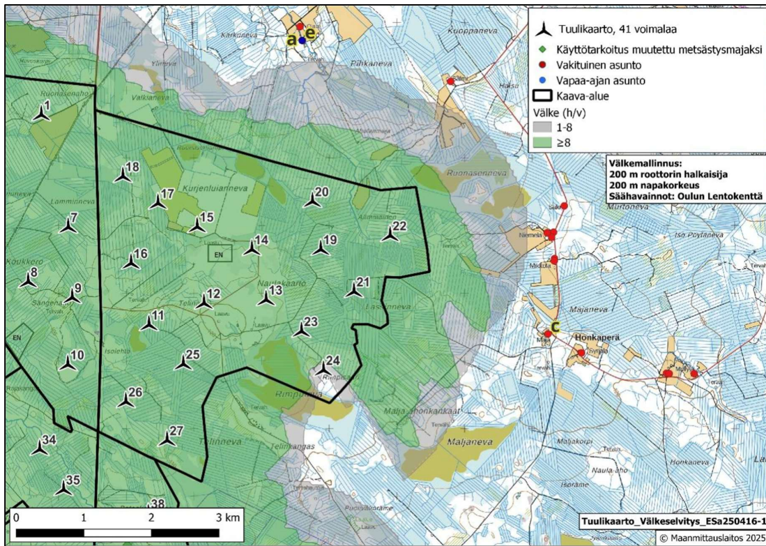
Kuva 78. Varjovälkkeen muodostuminen yhdessä Tuulikaarton muiden kaava-alueiden kanssa, Siikalatva itä kaava-alue.
