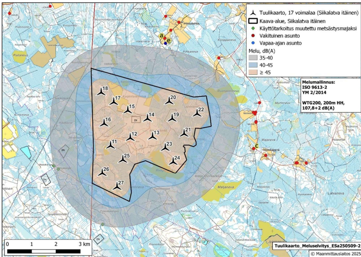
Kuva 52. Siikalatva itä -osayleiskaavan tuulivoimaloiden melumallinnus.
