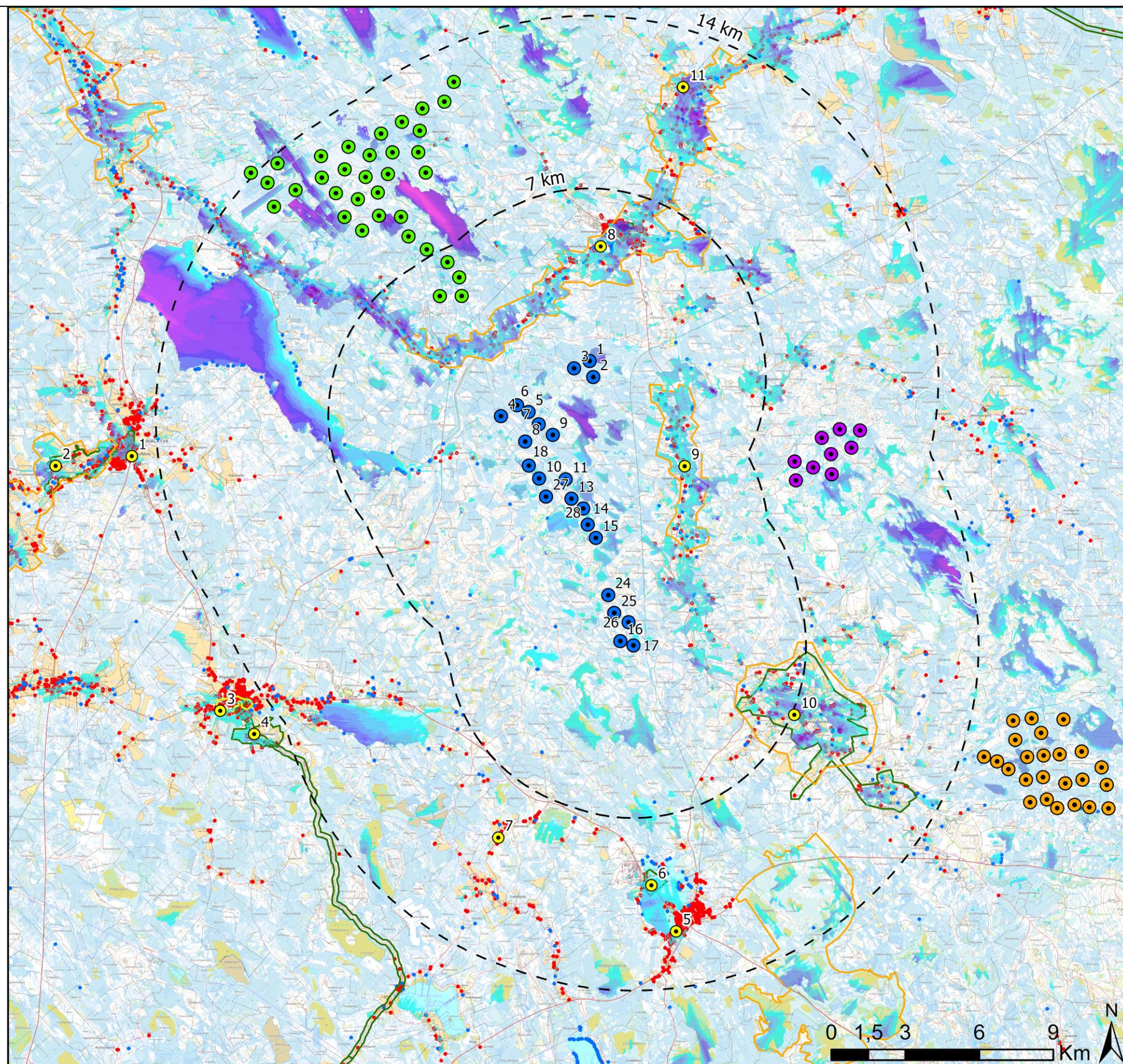
Kuva 2. Uljuan tuulivoimamahankkeen tuulivoimapaiston näkemäalueanalyysin laskentatulokset hankevaihtoehdossa VE 2 voimaloiden napakorkeudella mallinnettuna.
