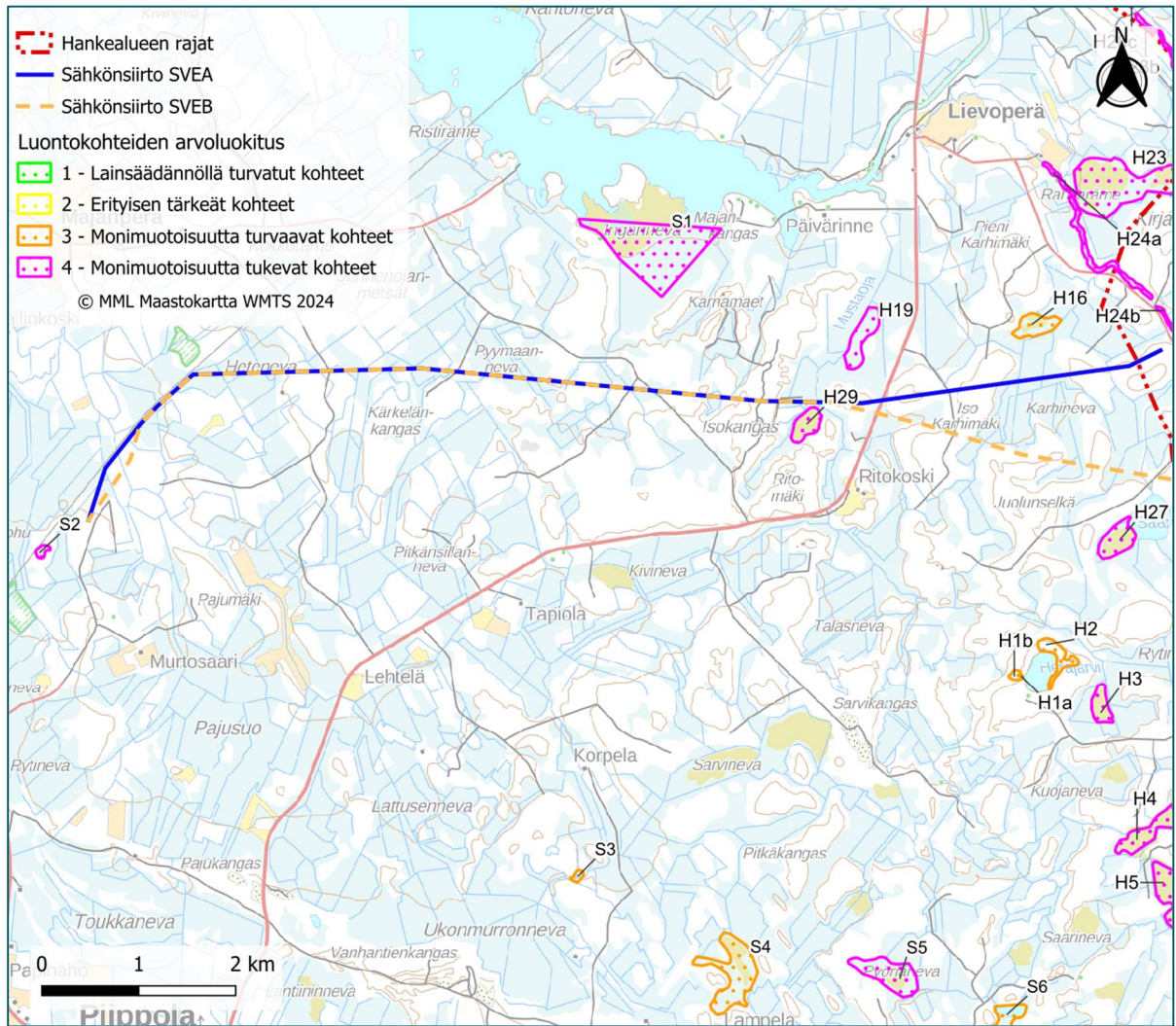
Kuva 26. Luontokohteiden sijainti sähkönsiirtoreiteillä. Numerointi vastaa alla luontokohteiden esittelyssä taulukossa 5 käytettyä numerointia.
