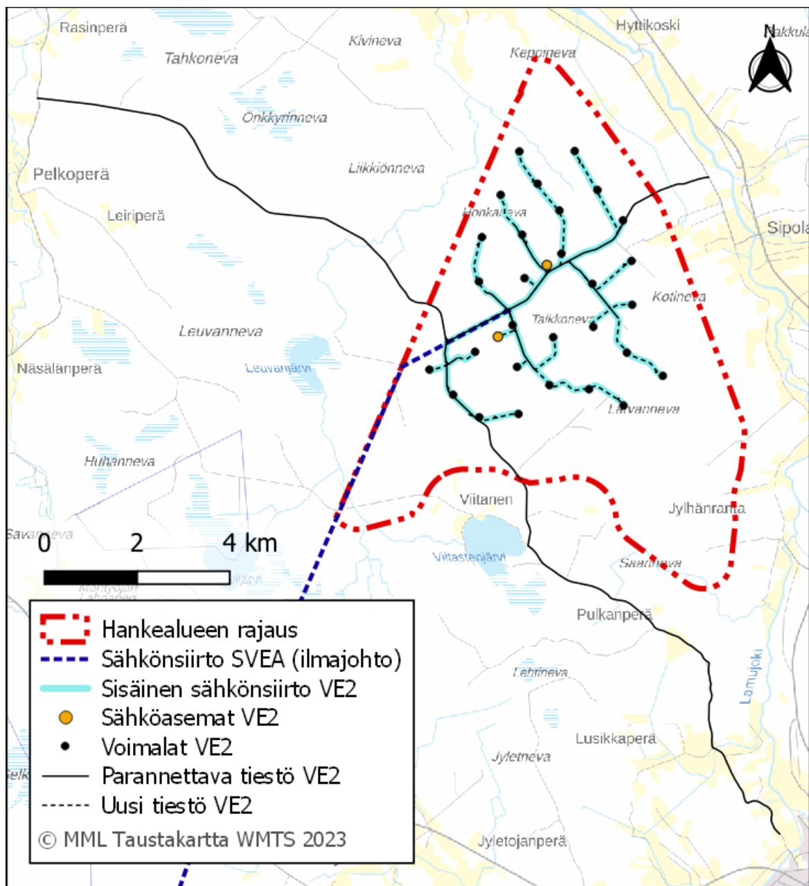
Kuva 3. Tuulivoima-alueen voimalasijoittelu hankevaihtoehdossa VE2. Yksi sisäntulotie parannetaan hankkeen toteutuessa (kartassa kaikki sisäntulotiet on osoitettu parannettavina).
